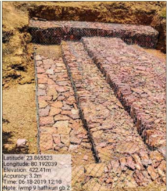
नदी पुनर्जीवन कार्यक्रम अंतर्गत लूज बोल्टर, गेबियन स्ट्रक्चर, कन्टूर ट्रेंच निर्माण कार्य जिला-खण्डवा
